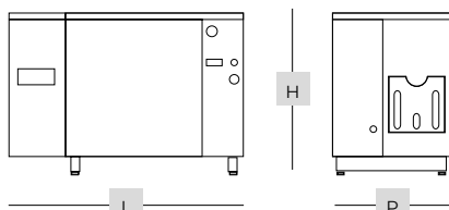
Modulo: compressore + essiccatore Module: compressor + dryer
