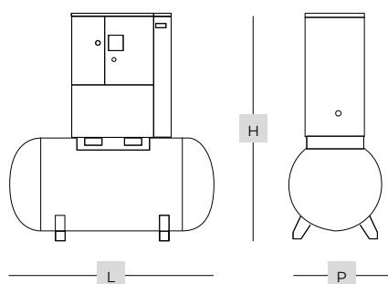
Modulo: compressore + serbatoio + essiccatore Module: compressor + tank + dryer
